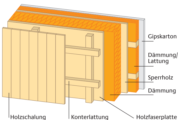
Holzrahmenbauweise
