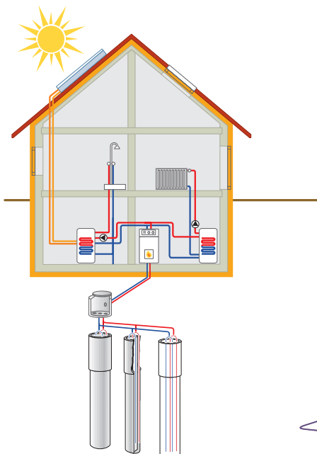
Wärmepumpe und Erdwärmesonden
