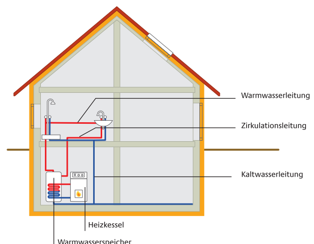
Zentrale Warmwasserversorgung
