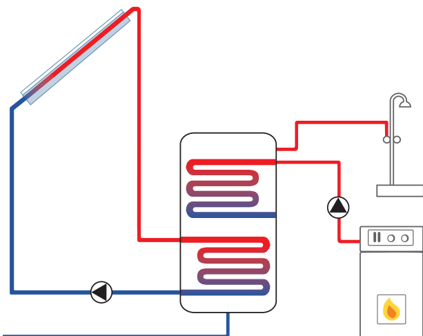
Funtionsschema Brennwerttechnik und Solaranlage
