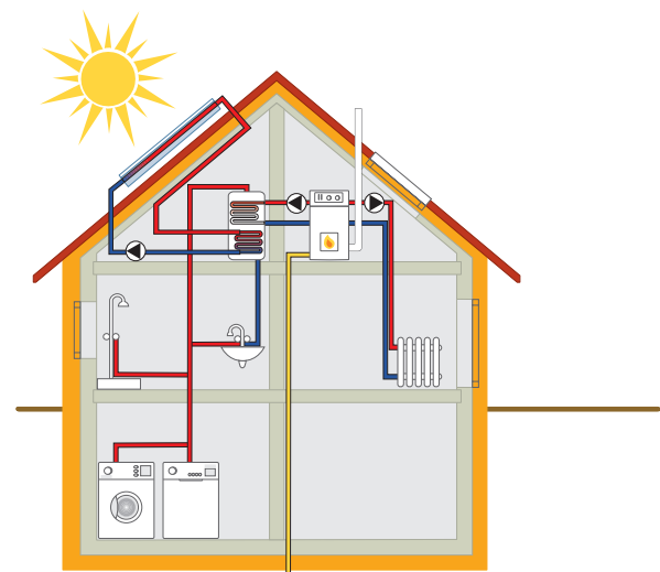
Funktionsschema einer solarthermischen Anlage
