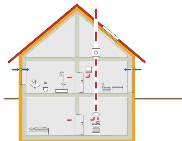
Abluftanlage
