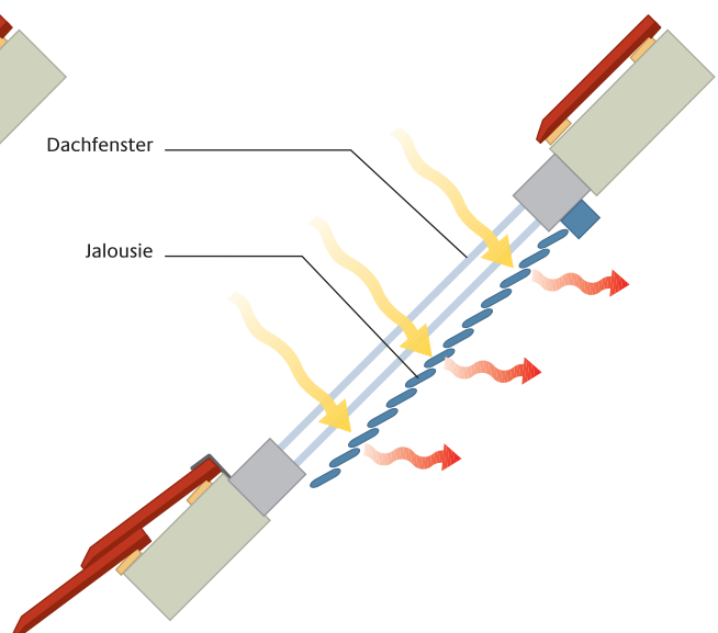
Sonnenschutz Jalousie innen: Wärme kommt herein
