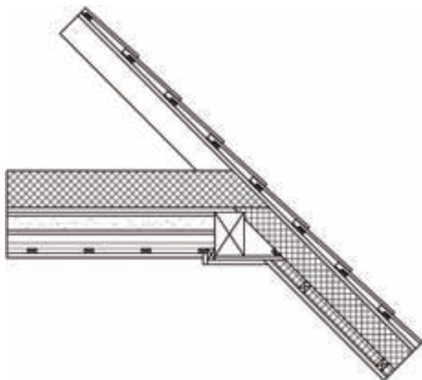
Wärmebrückenfreier Anschluss der Kehlbalke
