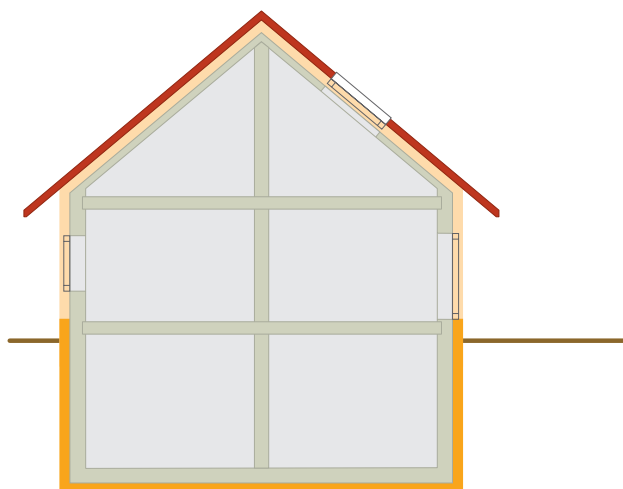
Dämmung Kellerwände und Bodenplatte
