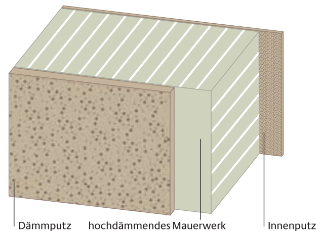
Monolithische Mauerwerkswand
