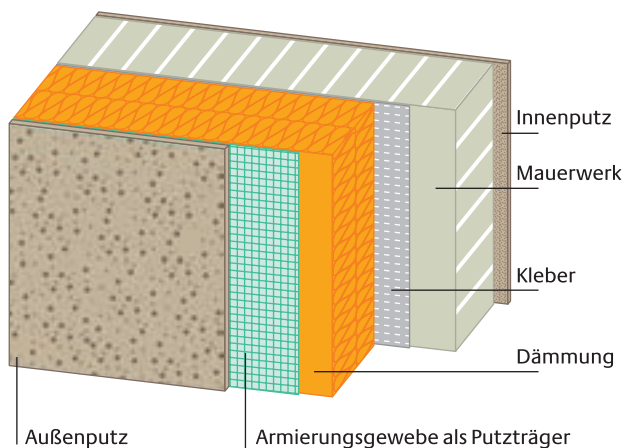
Wärmedämmverbundsystem
