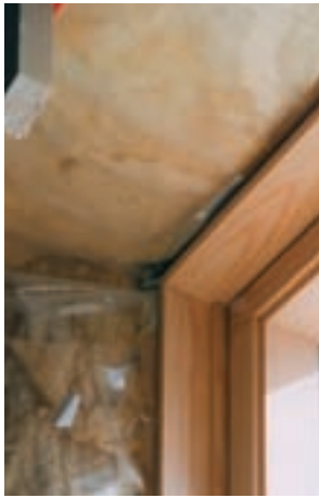
Luftdichter Anschluss eines Dachfensters mit Hilfe einer zugehörigen Schürze (Folie)
