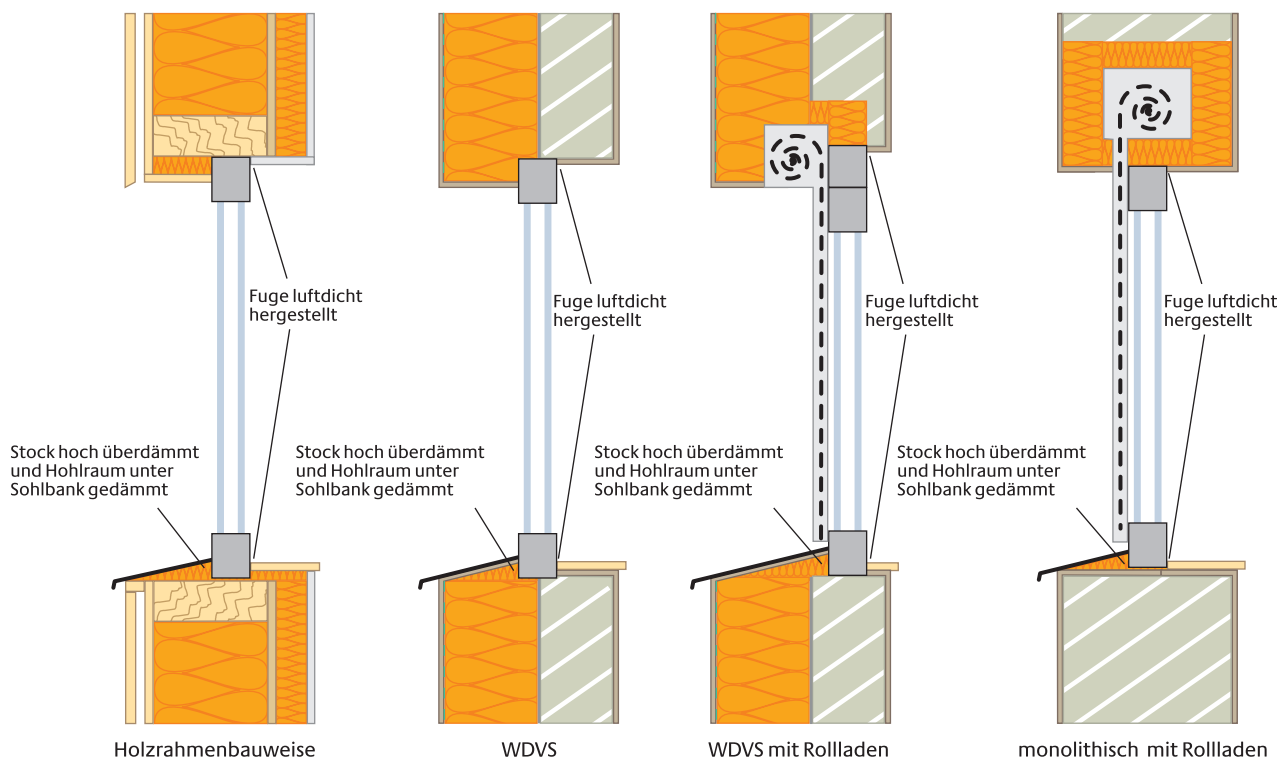
Einbausituation des Fensters bei verschiedenen Wandtypen
