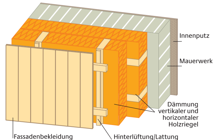
Vorhangfassade
